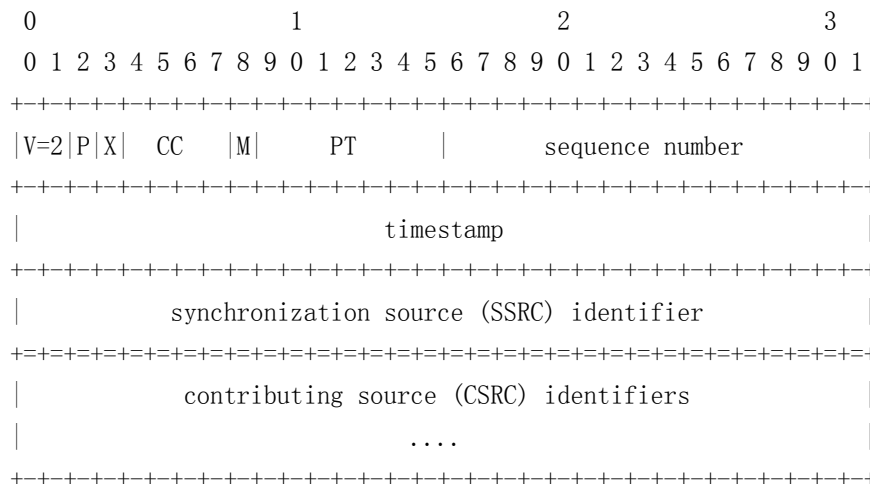
图 1. RTP 头。
