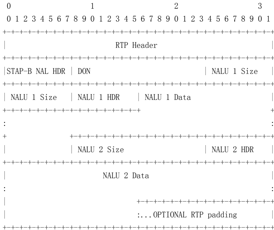
图 8. 一个RTP包包含一个STAP-B. STAP包含两个单时刻聚合单元例子
