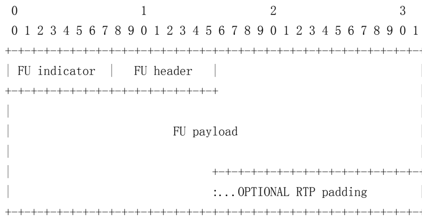
图 14. FU-A的RTP荷载格式
