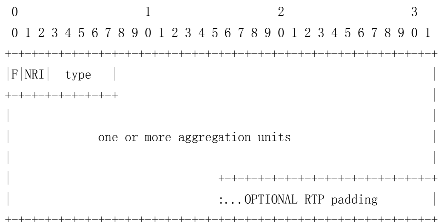
图 3. 聚合包的RTP荷载格式。
